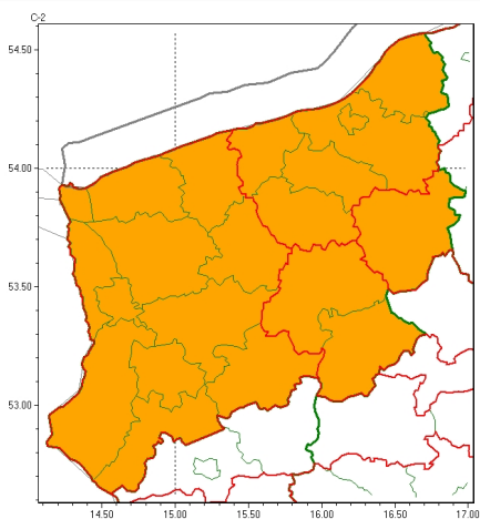
Opady marznące 2026-01-26 12:19
