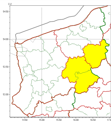
Gęsta mgła 2026-01-26 12:19
